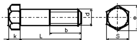
Болты с шестигранной головкой.
