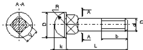
Болты с полукруглой головкой и квадратным подголовком. ГОСТ 7802-81
